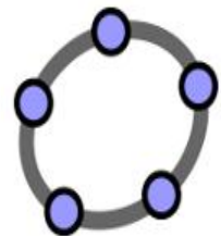
GeoGebra
